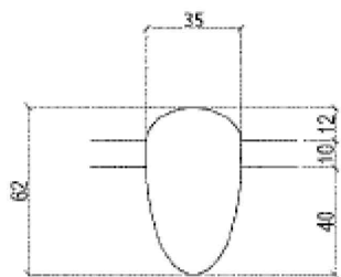
VUE DE FACE ERGOT ANTI - SKATE
