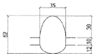
VUE EN PLAN ERGOT ANTI - SKATE
