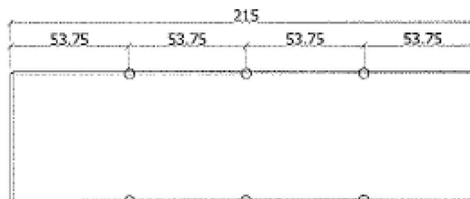
IMPLANTATION ERGOT ANTI-SKATE VUE EN PLAN BANQUETTE BA
