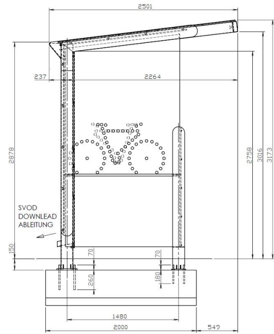
ZÁKLADOVÁ DESKA / FOUNDATION BASEPLATE / FUNDAMENTPLATTE 5000x2000x370 mm
