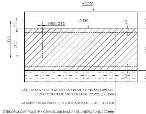
ZÁKLADOVÁ DESKA / FOUNDATION BASEPLATE / FUNDAMENTPLATTE 5000x2000x370 mm
