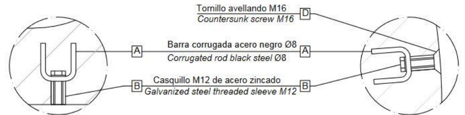
DETALLE N / DÉTAIL N
