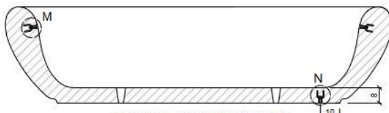
SECCIÓN A-A' / SECTION A-A'
